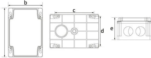
الرسم الفني
