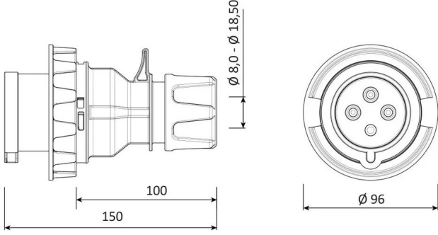
الرسم الفني
