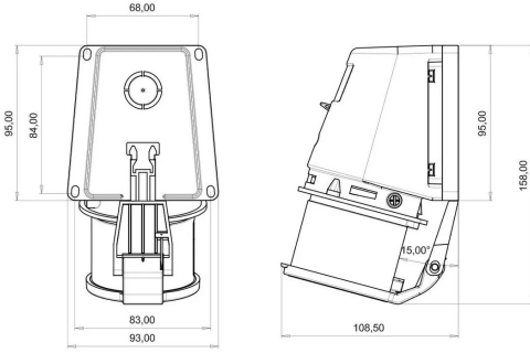
الرسم الفني
