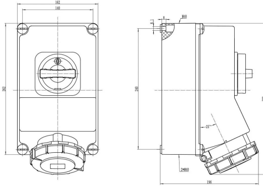
الرسم الفني
