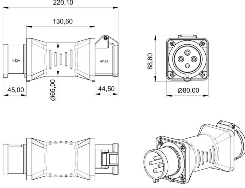
الرسم الفني
