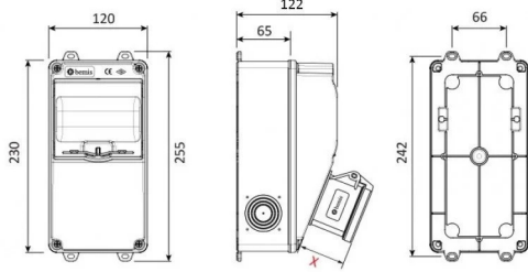
الرسم الفني
