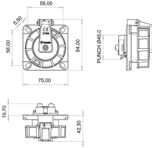
الرسم الفني
