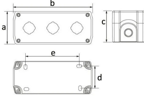
Ölçüler / Dimensions (mm)
