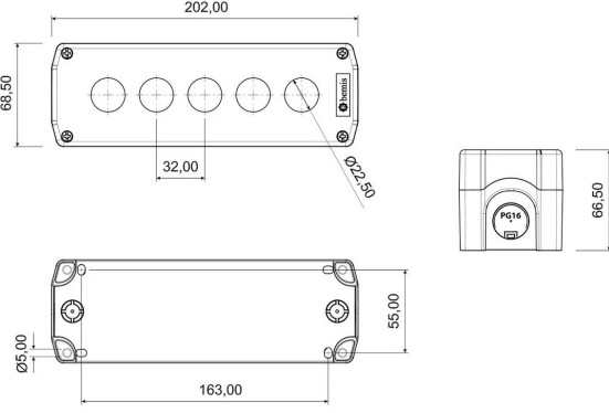
الرسم الفني
