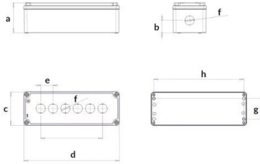
Ölçüler / Dimensions (mm)
