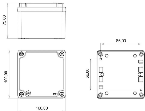
الرسم الفني
