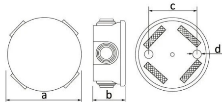
Ölçüler / Dimensions (mm)
