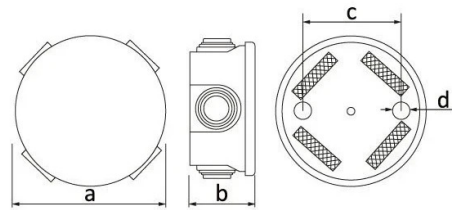
MASSZEICHNUNG
