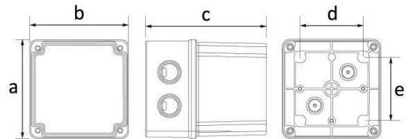
MASSZEICHNUNG
