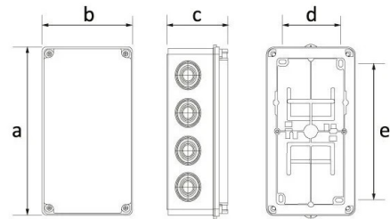
Ölçüler / Dimensions (mm)
