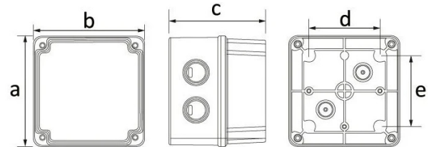
MASSZEICHNUNG
