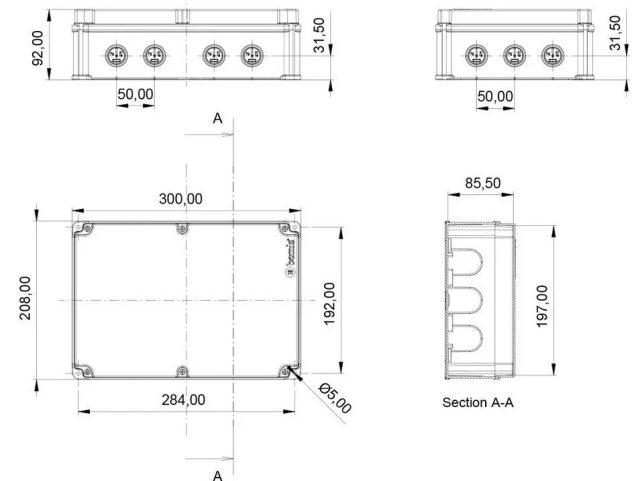
MASSZEICHNUNG
