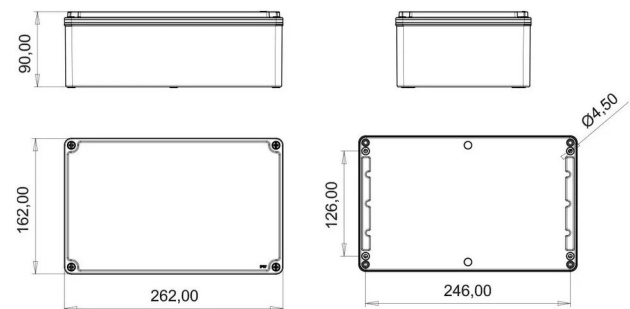
MASSZEICHNUNG
