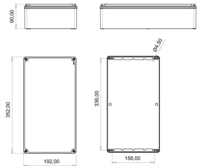
MASSZEICHNUNG
