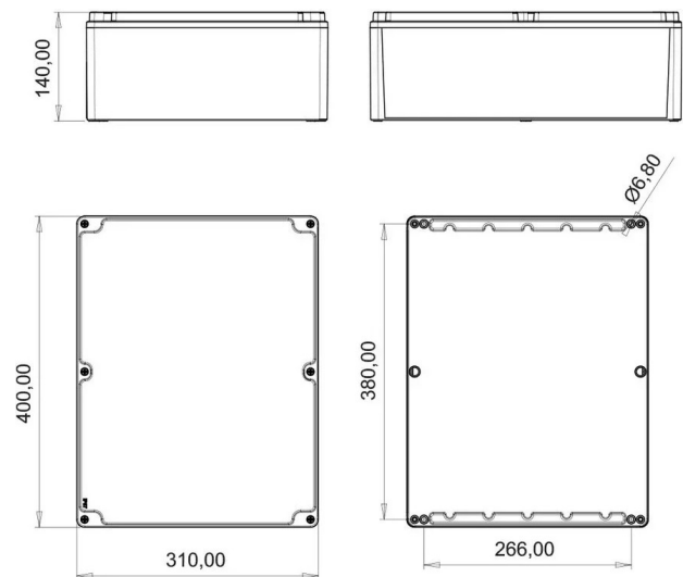
MASSZEICHNUNG
