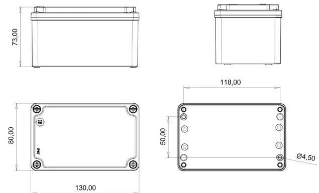
MASSZEICHNUNG
