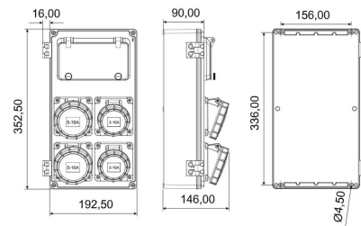
MASSZEICHNUNG
