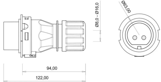
MASSZEICHNUNG
