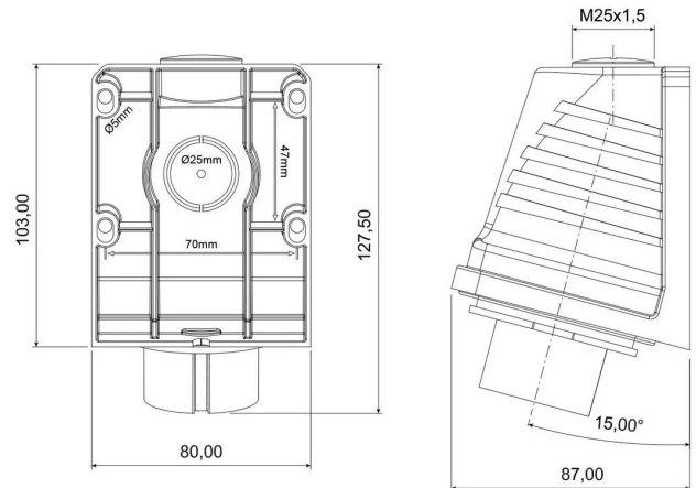
MASSZEICHNUNG
