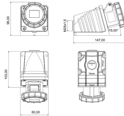
MASSZEICHNUNG
