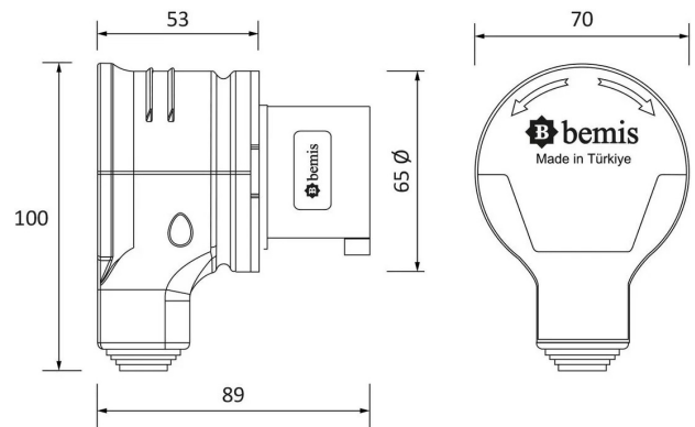
MASSZEICHNUNG
