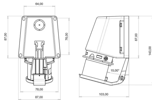
MASSZEICHNUNG
