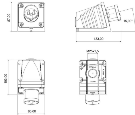
MASSZEICHNUNG
