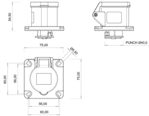
MASSZEICHNUNG
