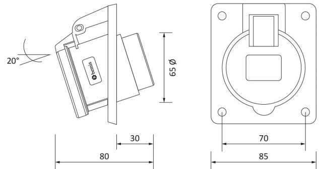
MASSZEICHNUNG
