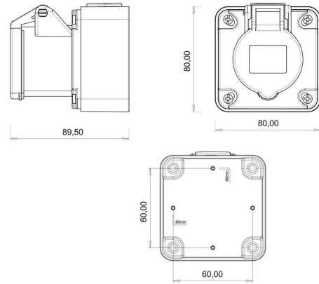
MASSZEICHNUNG
