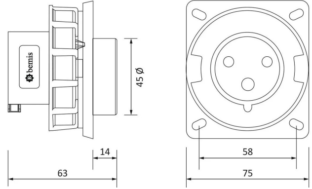
MASSZEICHNUNG
