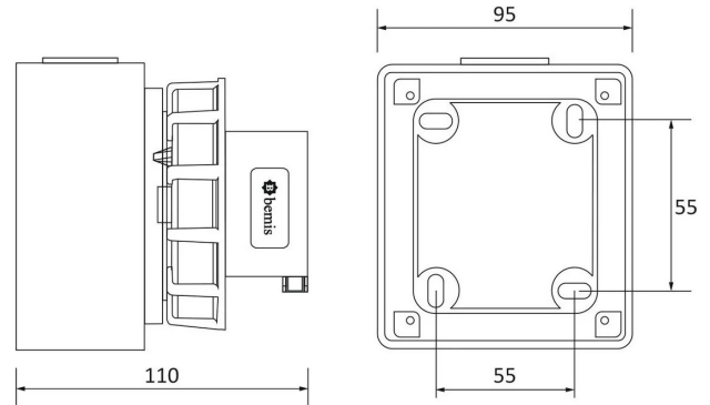
MASSZEICHNUNG
