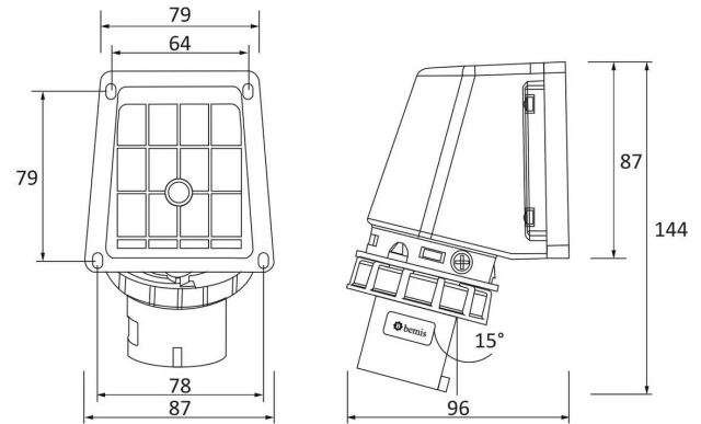
MASSZEICHNUNG
