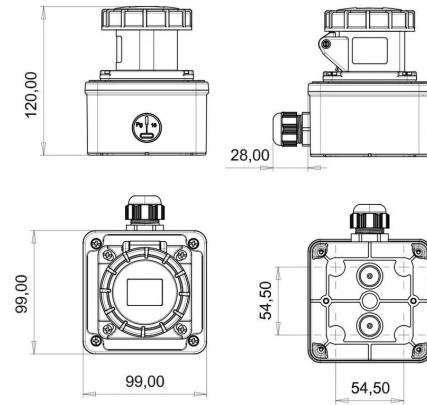
MASSZEICHNUNG
