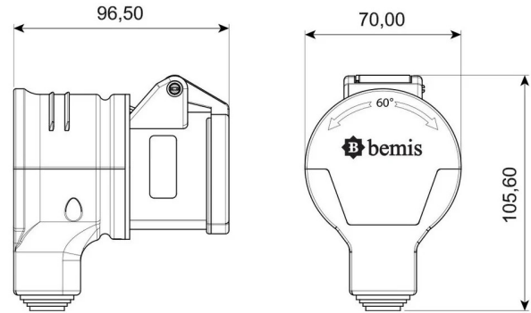
MASSZEICHNUNG
