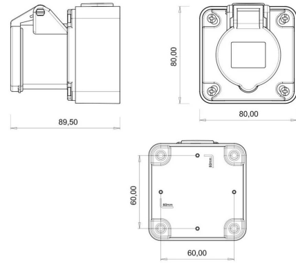
MASSZEICHNUNG
