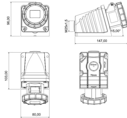
MASSZEICHNUNG
