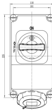
MASSZEICHNUNG
