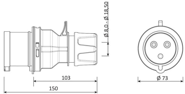
MASSZEICHNUNG
