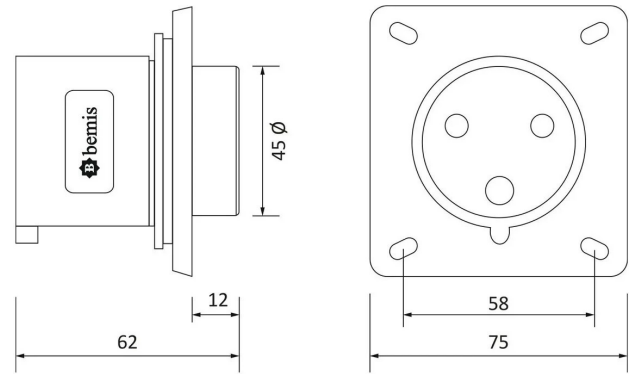
MASSZEICHNUNG
