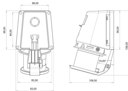
MASSZEICHNUNG
