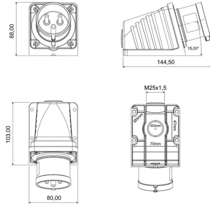
MASSZEICHNUNG
