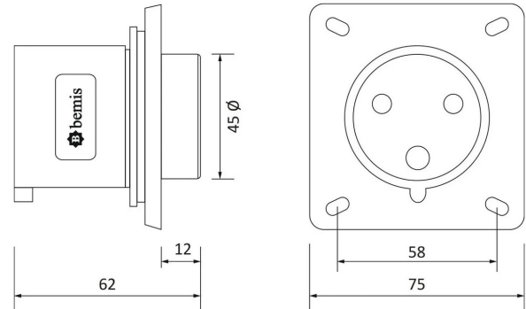
MASSZEICHNUNG
