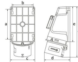
Ölçüler / Dimensions (mm)
