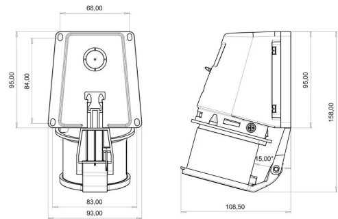
MASSZEICHNUNG
