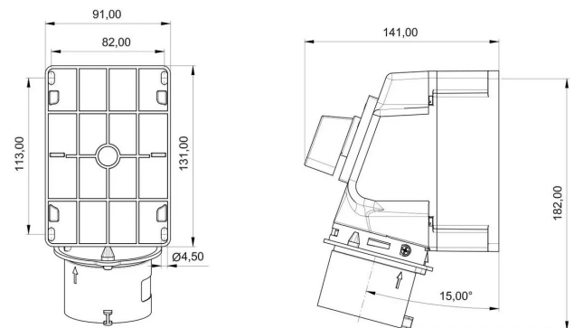
MASSZEICHNUNG
