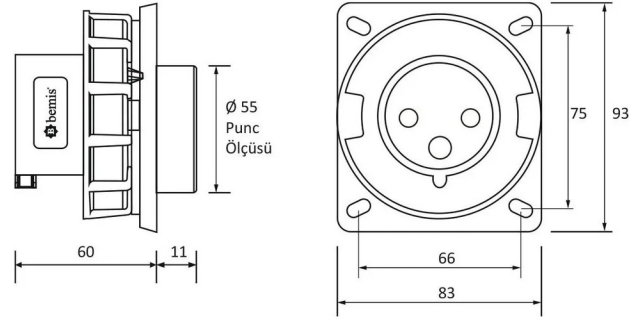
MASSZEICHNUNG
