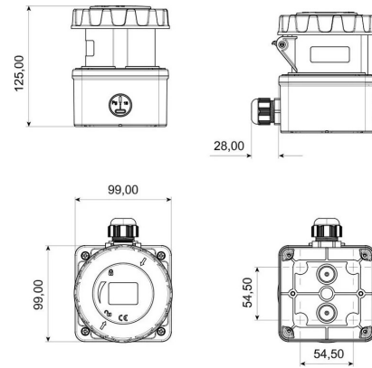
MASSZEICHNUNG
