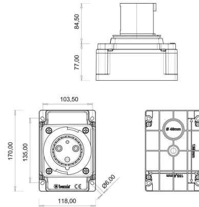
MASSZEICHNUNG
